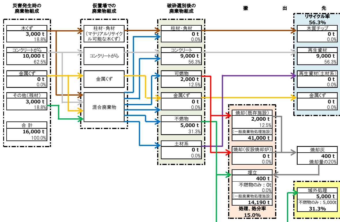
図 2-8 高山・大原断層帯地震における災害廃棄物処理フロー
