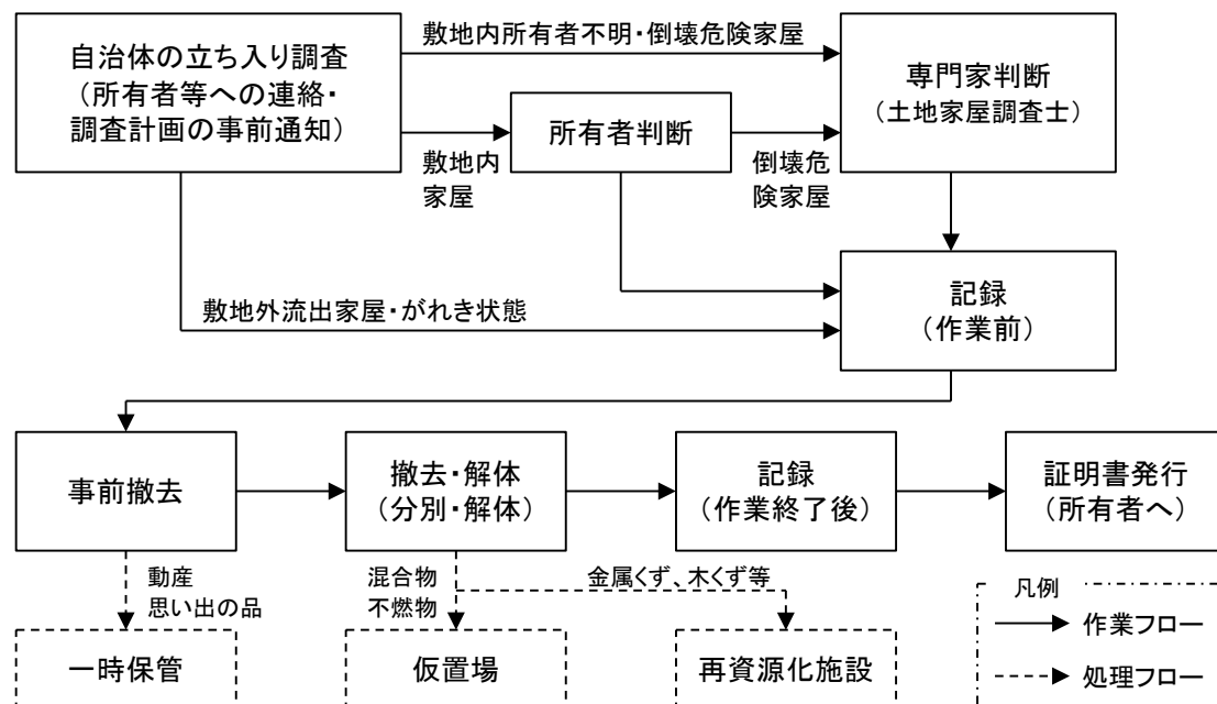
図 2-11 解体・撤去の作業及び処理フロー
