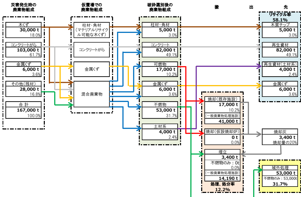
図 2-6 養老一桑名一四日市断層帯地震における災害廃棄物処理フロー
