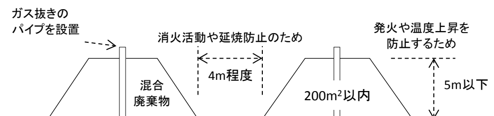
図 2-3 混合仮置場模式図
