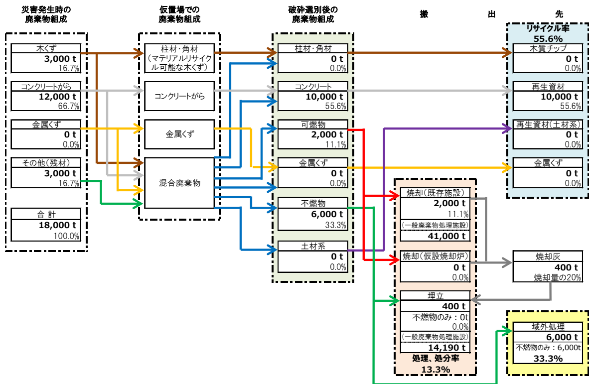
図 2-7 阿寺断層系地震における災害廃棄物処理フロー
