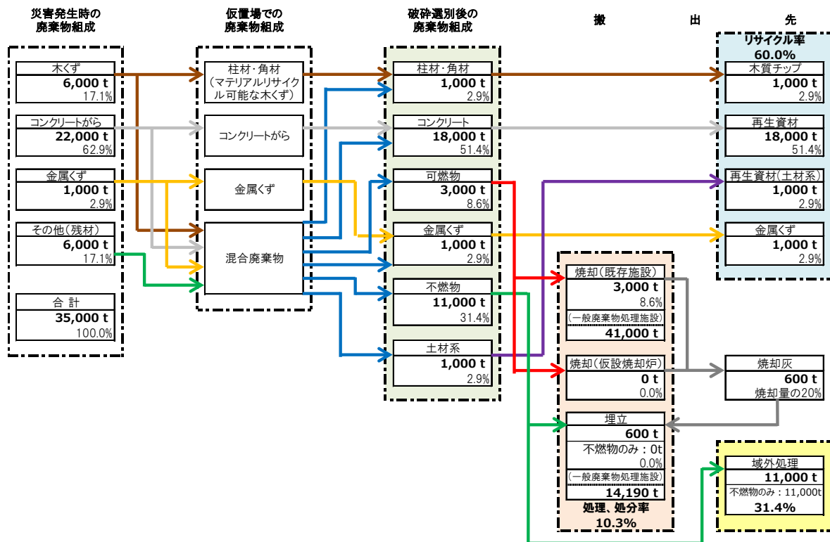
図 2-9 跡津川断層帯地震における災害廃棄物処理フロー
