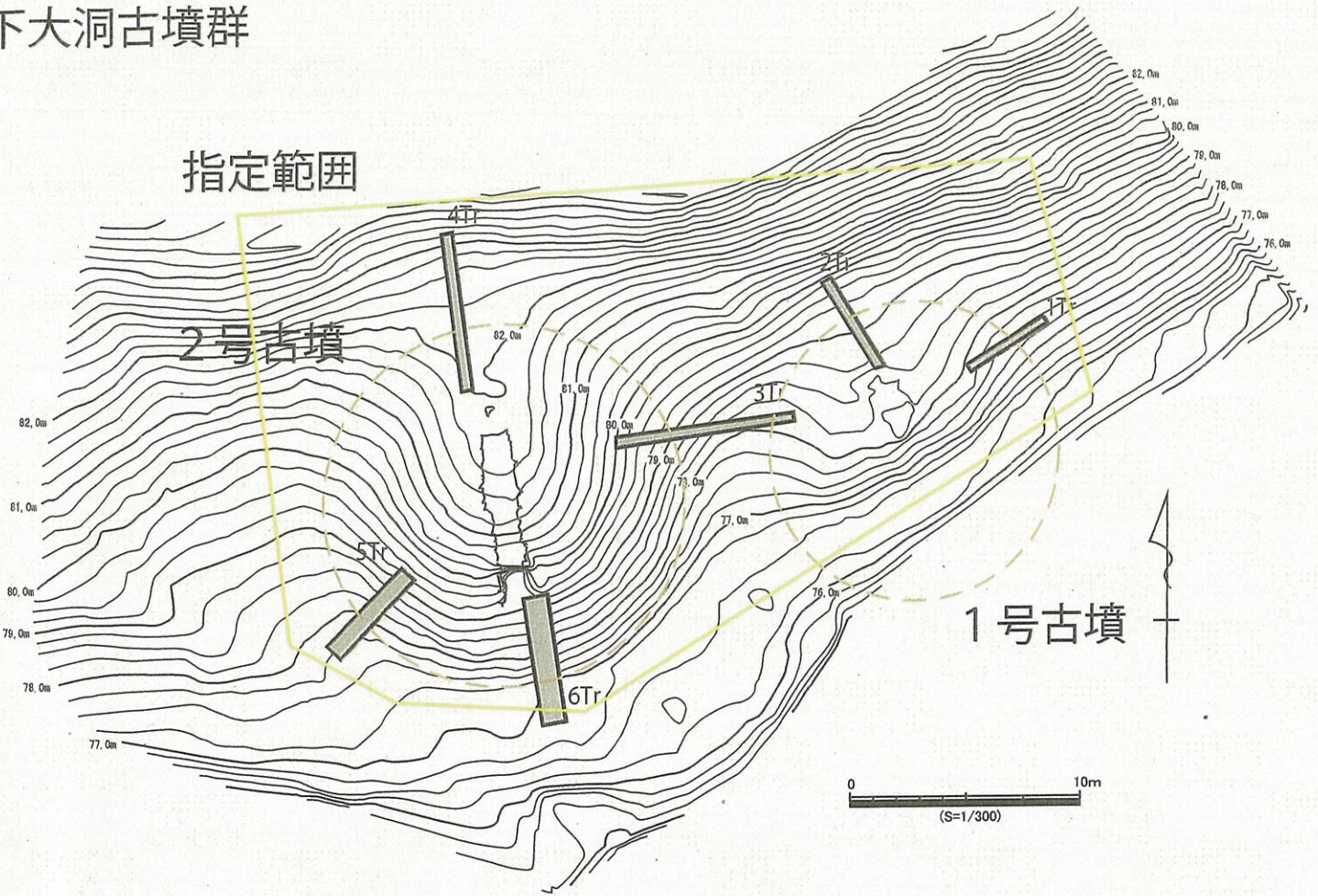
墳丘測量図
