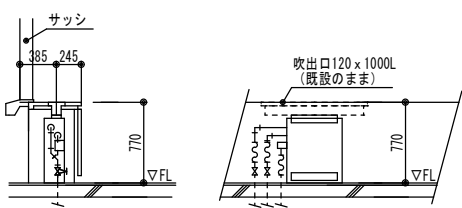
床置埋込ファンコイル廻り納まり図
